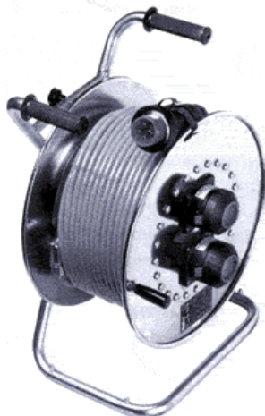
Переносной распределитель розеток с катушкой
