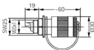
Фланцевый штекер
