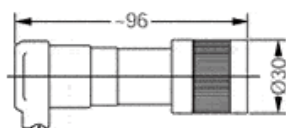
Штекер
