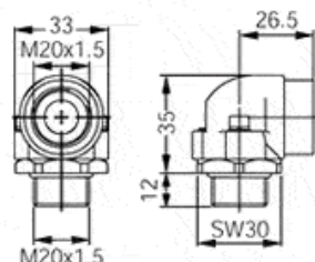
Угольник
