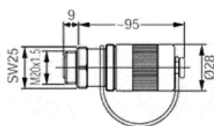
Фланцевая розетка
