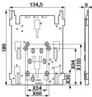
Крепление на стене
