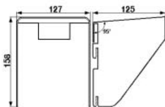
Защитная крышка, размер 1
