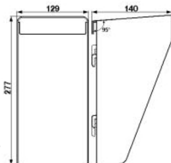
Защитная крышка, размер 4
