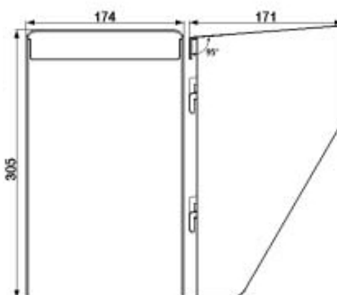
Защитная крышка, размер 5
