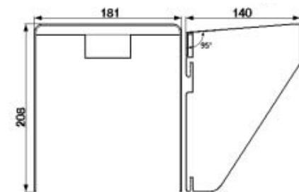
Защитная крышка, размер 2A
