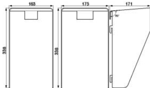
Защитная крышка, размер 3, для вертикальных элементов (размер 3)
