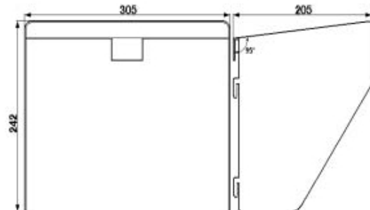
Защитная крышка, размер 3, для горизонтальных элементов (размер 3)
