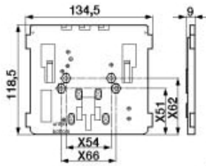
Крепление на стене
