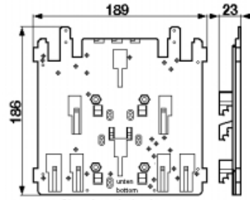
Крепление на решетке
