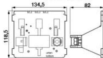
Крепление на трубах
