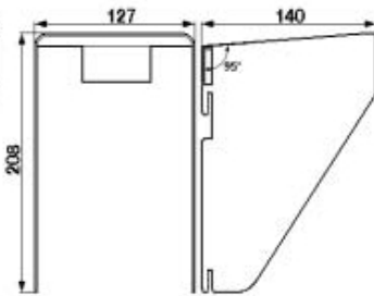
Защитная крышка, размер 2
