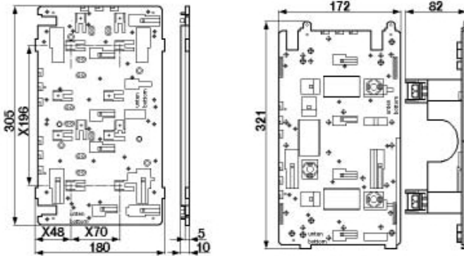
Элемент монтажа, размер 3, вертикальный, для крепления на стене, решетке и трубах
