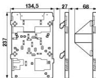
Элемент монтажа, размер 4, для крепления на стене, решетке и трубах
