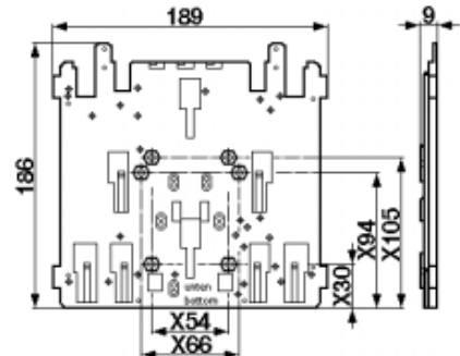
Крепление на стене
