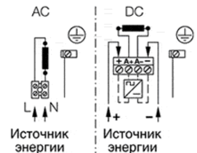
Схема подключения зажимов
